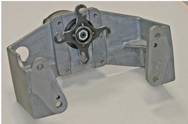
Hydraulikpumpenantrieb für Traktoren
