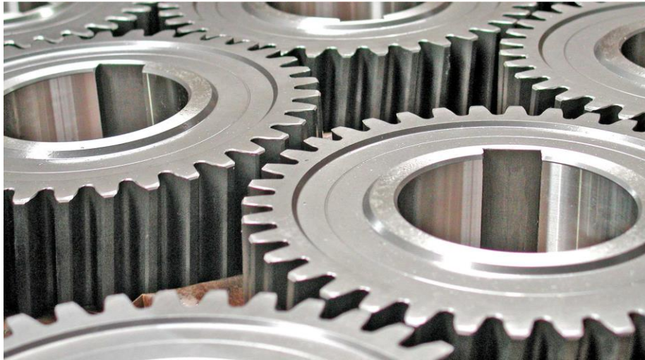
Kupplungselemente für Traktor-Schaltgetriebe, innen und außen, konisch gestoßen
